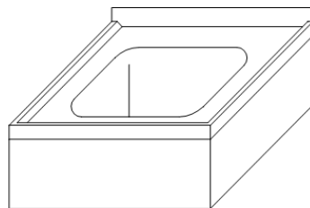
Kmora o wymiarze 400x400x250 mm
