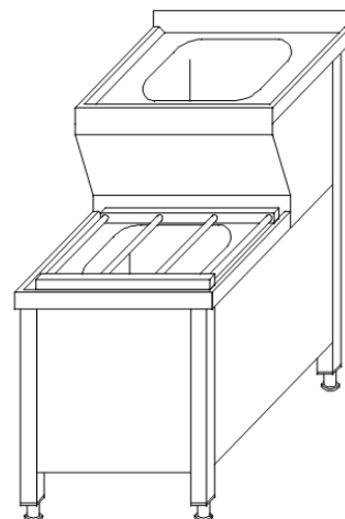
Dwie komory o wymiarze 340x300x180 mm każda
